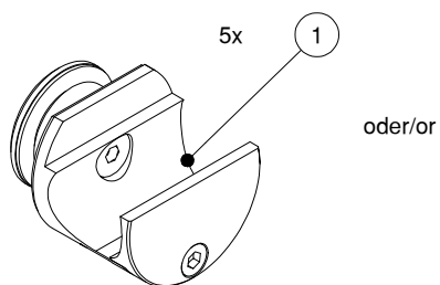
Klemmhalter an Glas, mit aufliegenden oder versenkten Punkthalter
